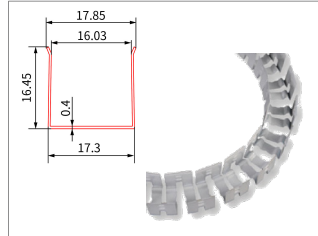
8767000003 - Calha Inox Flex. (Rolo1000mm)
