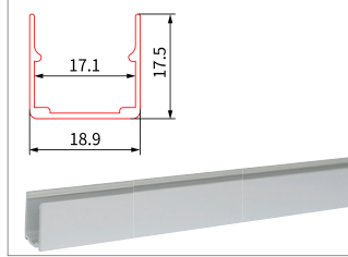
8767000002 - Calha Aluminio (1000mm)
